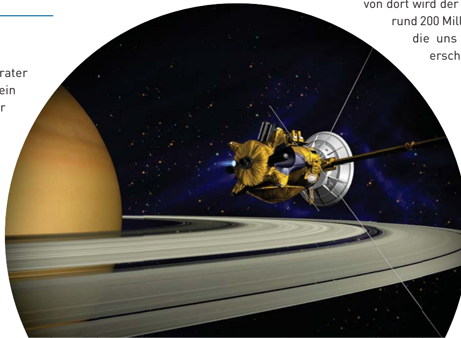
Cassini-Orbiter – Raumsonde zur Erforschung des Planeten Saturn Bild: NASA
