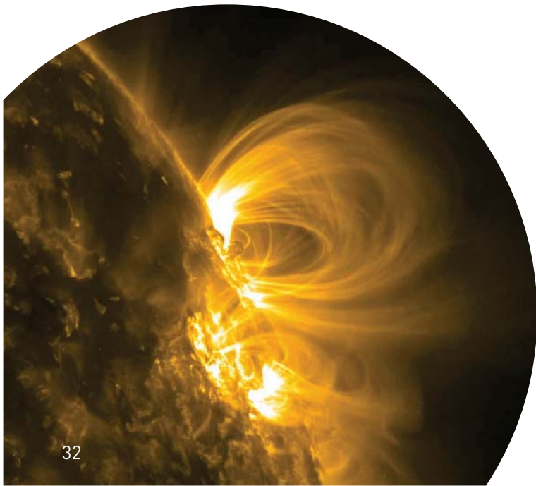
Sonnenexplosion / Bild: NASA/SDO.
